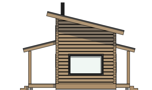
Julkisivu länteen 1:100
