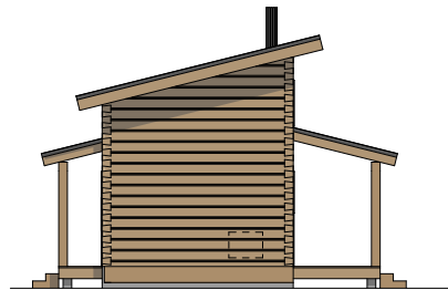
Julkisivu itään 1:100
