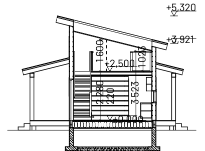
Leikkaus A - A 1:100
