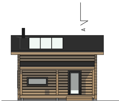
Julkisivu etelään 1:100
