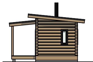
Julkisivu itään 1:100
