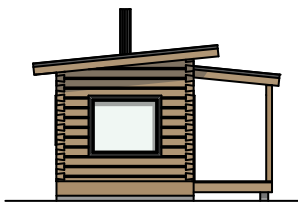
Julkisivu länteen 1:100
