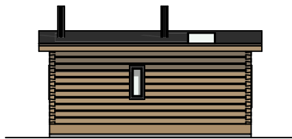
Julkisivu pohjoiseen 1:100
