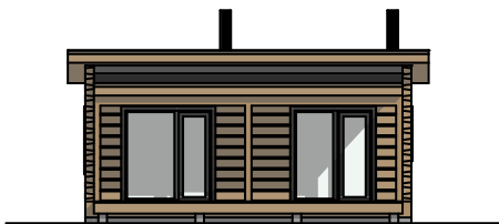
Julkisivu etelään 1:100
